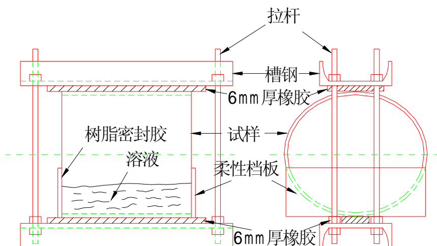
图 B1 长期弯曲应变试验装置
